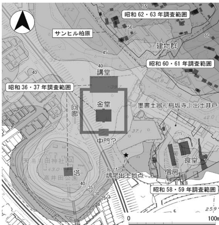
▲鳥坂寺跡全体図
