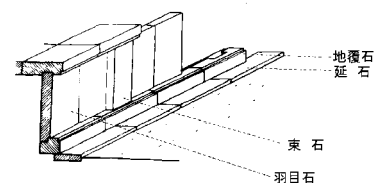
基壇と延石
