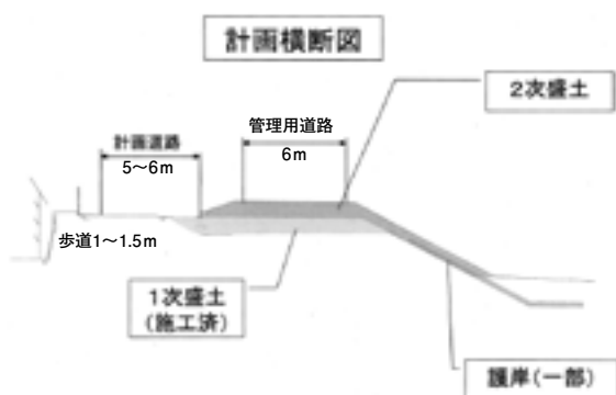
計画道路横断面図
