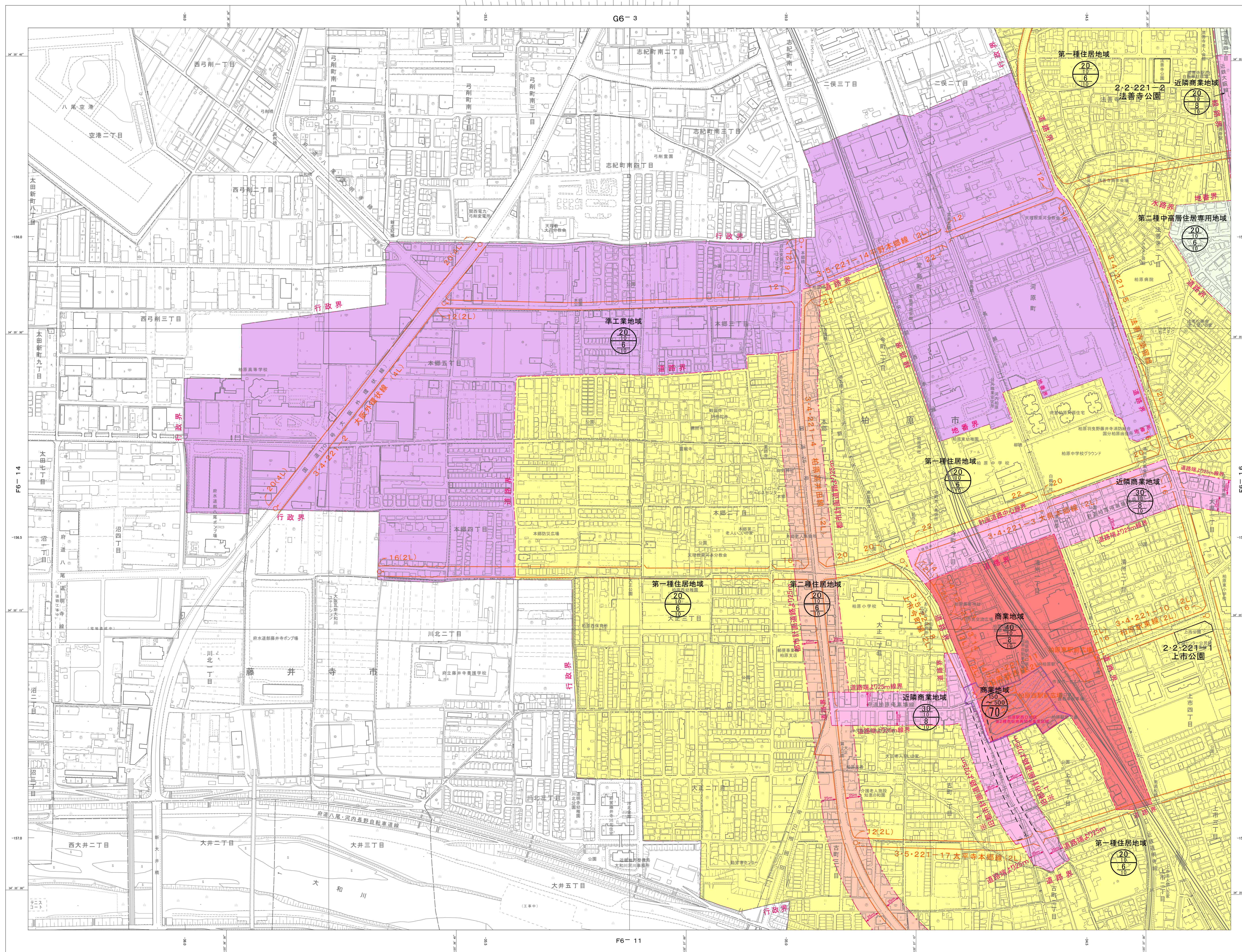
概観図(大F-6-15)
