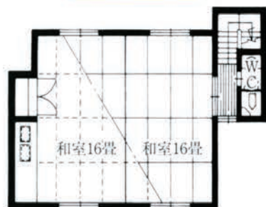
2階平面図
