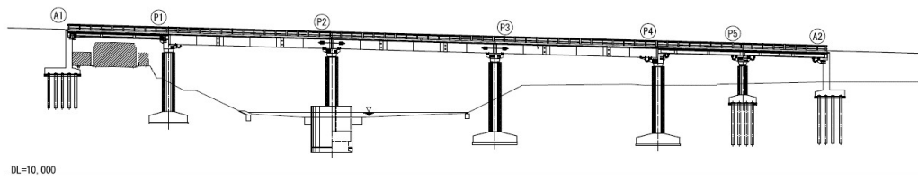
側面図
