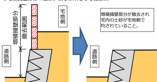
○増積擁壁部分の図解、及び解消となる撤去例
