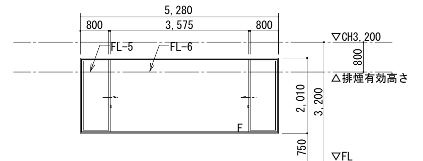
改修後 1階建具表 S=1/100
