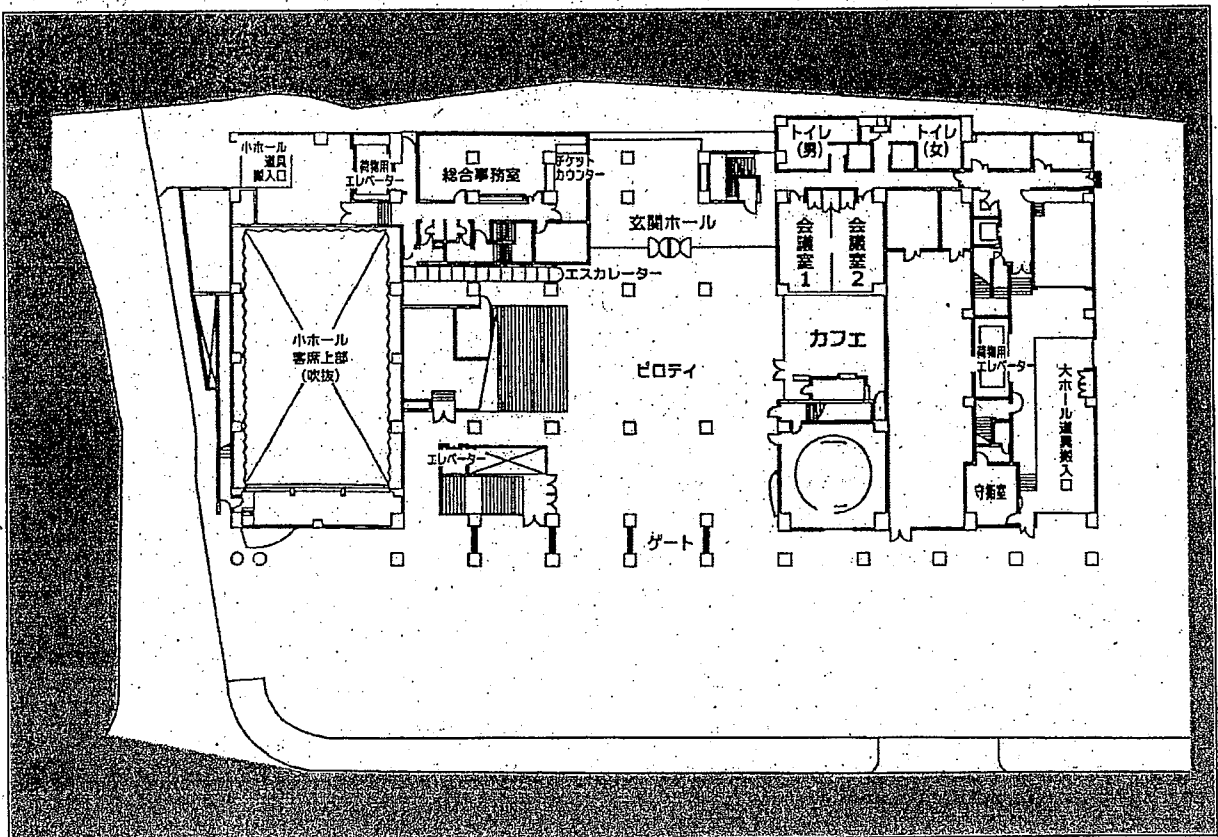
1階平面図
